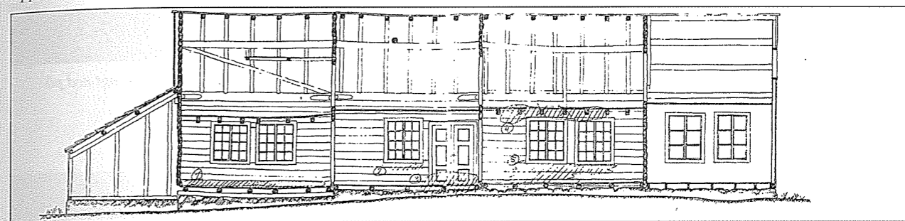
Over: Snitt gjennom skut, bu, gang, stove og endekammers. Under: Grunnplan av 1. etasje.
