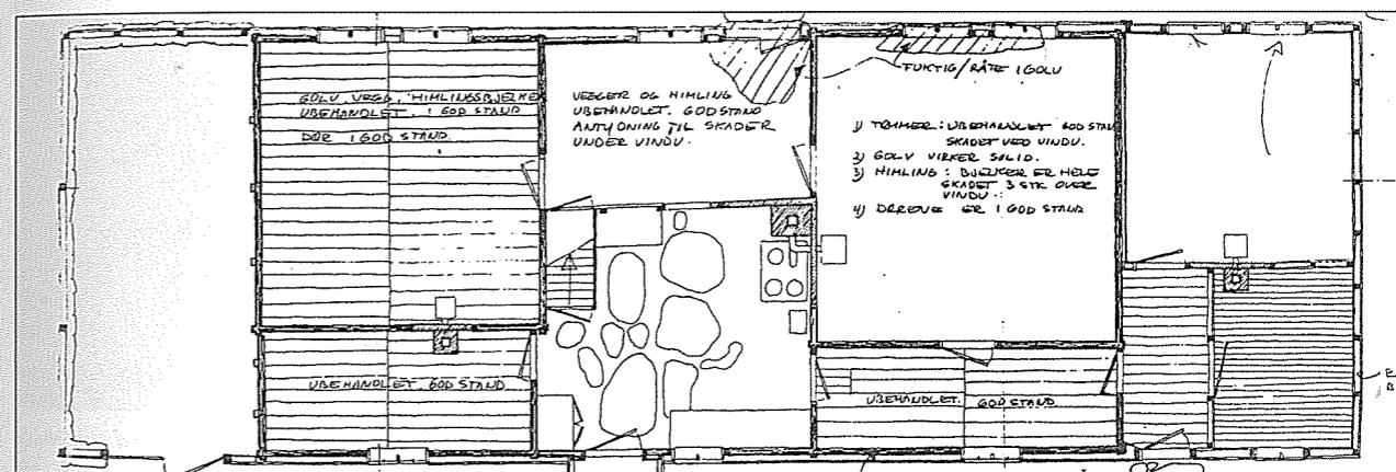
Over: Snitt gjennom skut, bu, gang, stove og endekammers. Under: Grunnplan av 1. etasje.
