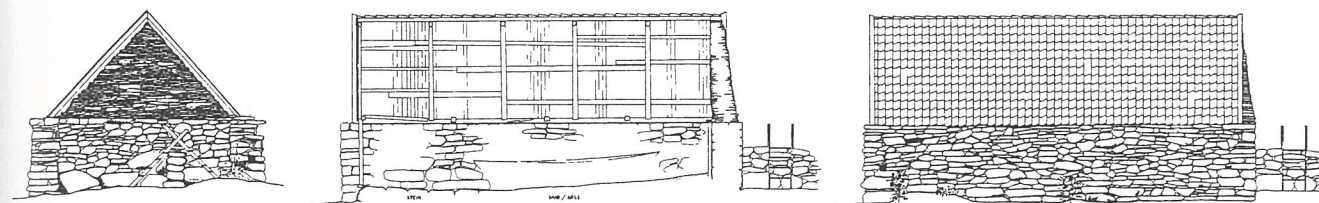
Oppmålingstegninger av gammelt steinnaust på Vistnes lenger sør i Randaberg. Miljøprosjektet. Hilde Schjelderup, Solbjørg Sandve, Åse Kvalvik.
