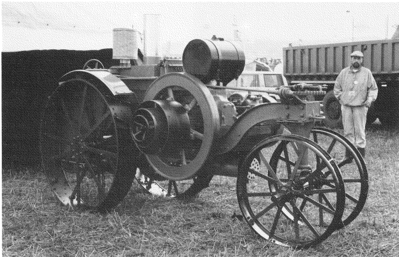
Traktoren Mogul 10–20 blei vist fram første gang på Pløye-VM i Klepp hausten 1989. Styremedlem Hans Voll la tilrette både for Jærmuseet si utstilling og for programmet vårt: «Frå Spade til vendepløg.» Foto: Jærmuseet
