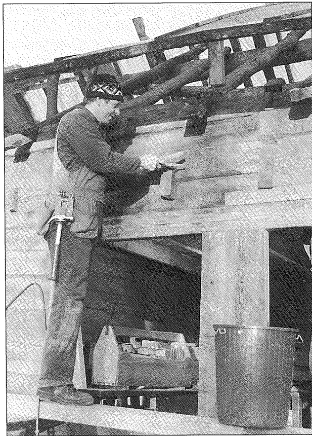
Byggmester Trond Nærland i arbeid på Audamotland. Foto: Jærmuseet
